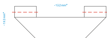
sposób wszywania etykiet tkanych typu wieszaczek zwykły
