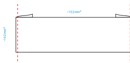
sposób wszywania etykiet tkanych z podwinięciami
