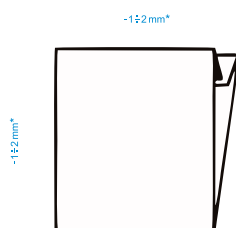
sposób wszywania etykiet tkanych składanych na pół „typu book cover”
